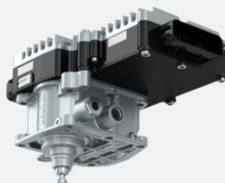
PEÇAS MÓDULO GS (HW04/06)
